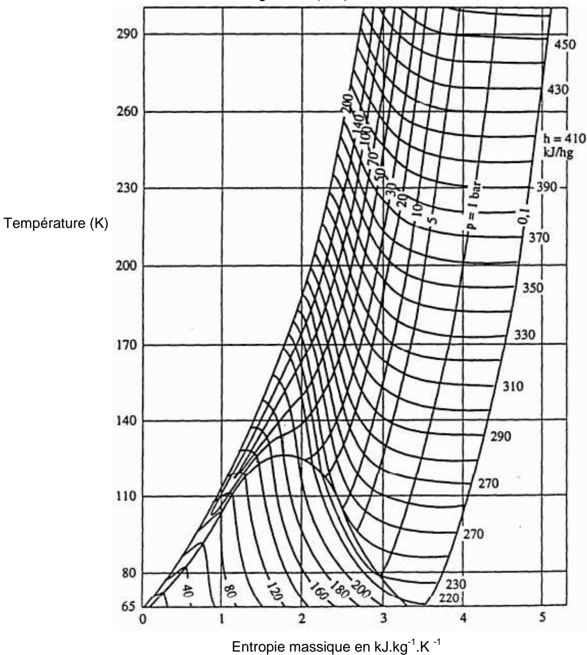
Diagramme (T, s) du diazote
